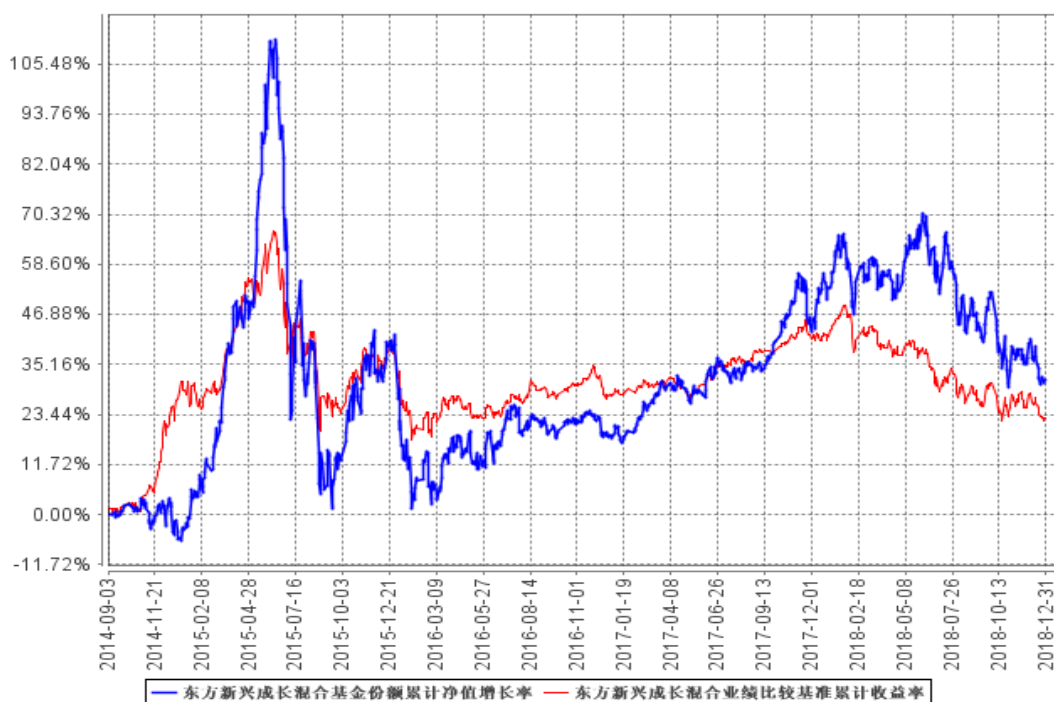
东方新兴成长混合基金份额累计净值增长率与同期业绩比较基准收益率的历史走势对比图
